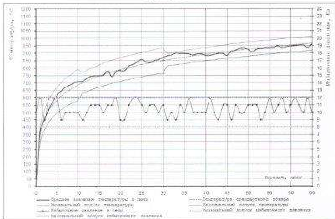
Рис. 4. Изменение температурного режима в камере печи.
