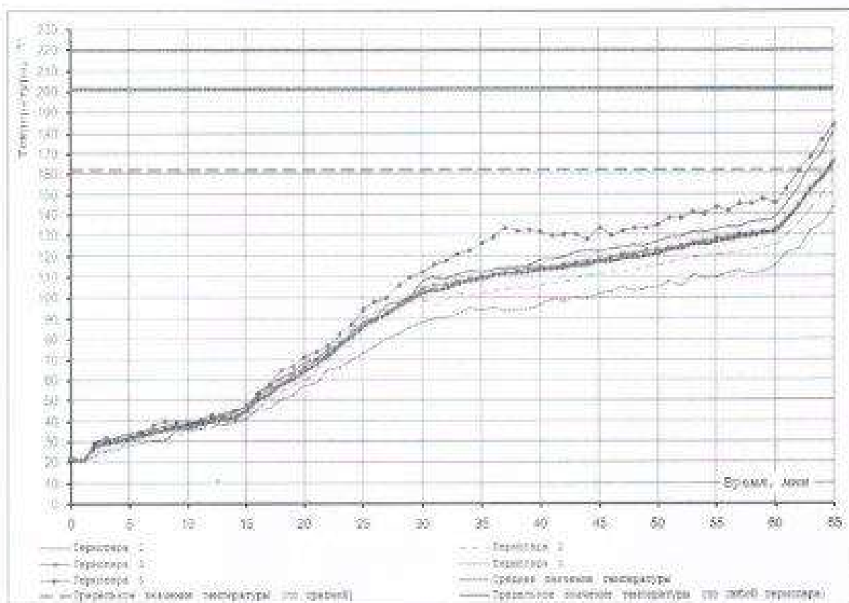
Рис. 5. Изменения температуры на необогреваемой поверхности образца.
