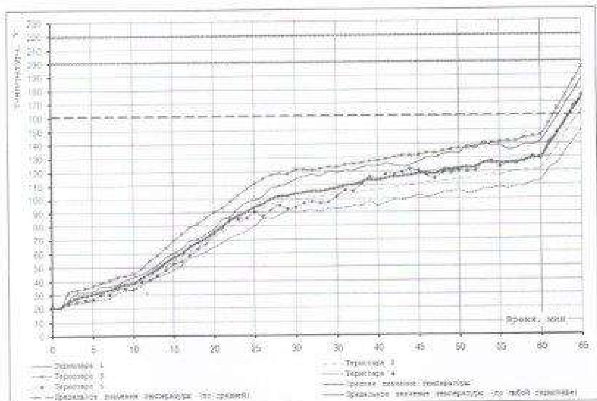
Рис. 3. Изменение температуры на необогреваемой поверхности образца.
