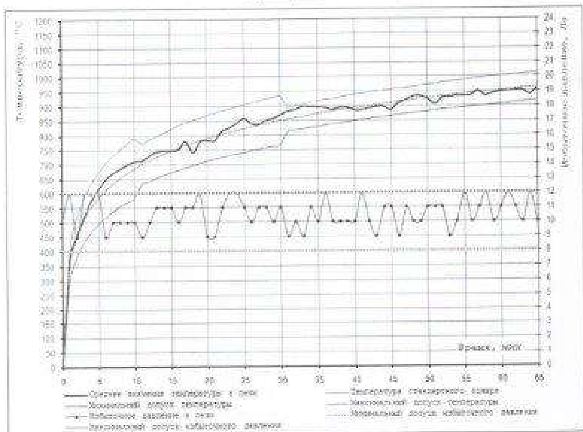
Рис. 2. Изменение температурного режима в острой камере печи.
